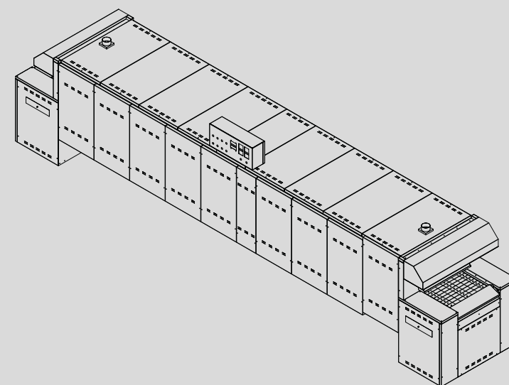
ALTEZZA CAMERA DI COTTURA 85 mm HEIGHT OF COOKING CHAMBER 85 mm
